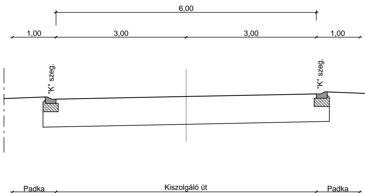
F-F metszet, magánút közforgalom számára megnyitott
